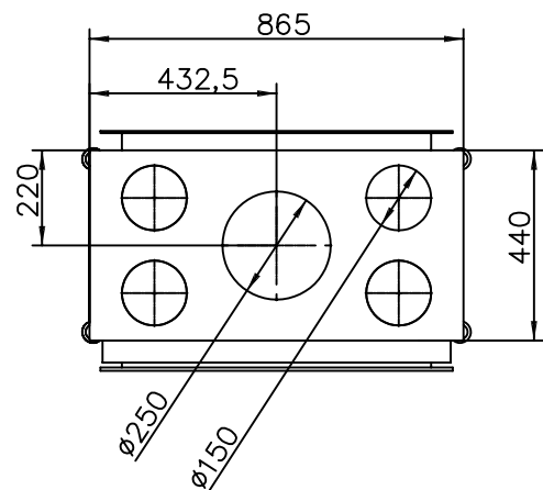
Bovenaanzicht Draufsicht Echangeur Top view
