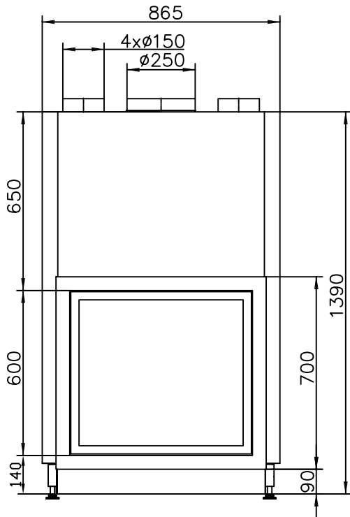
Vooranzicht Frontansicht Vue de face Front view
